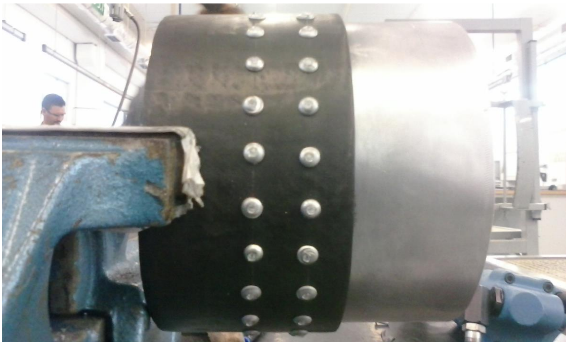
FOTO 3 – Rebites a Remover marcados com Punção (Exercício Avaliação)
