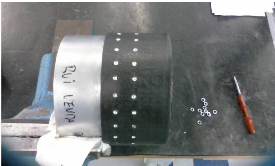
FOTO 5 – Cabeças dos Rebites Removidas (Exercício Avaliação)
