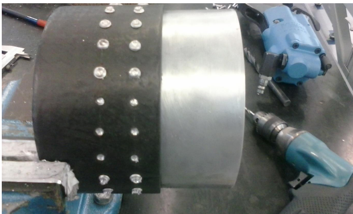
FOTO 4 – Remoção da Cabeça do Rebite (Exercício Avaliação)
