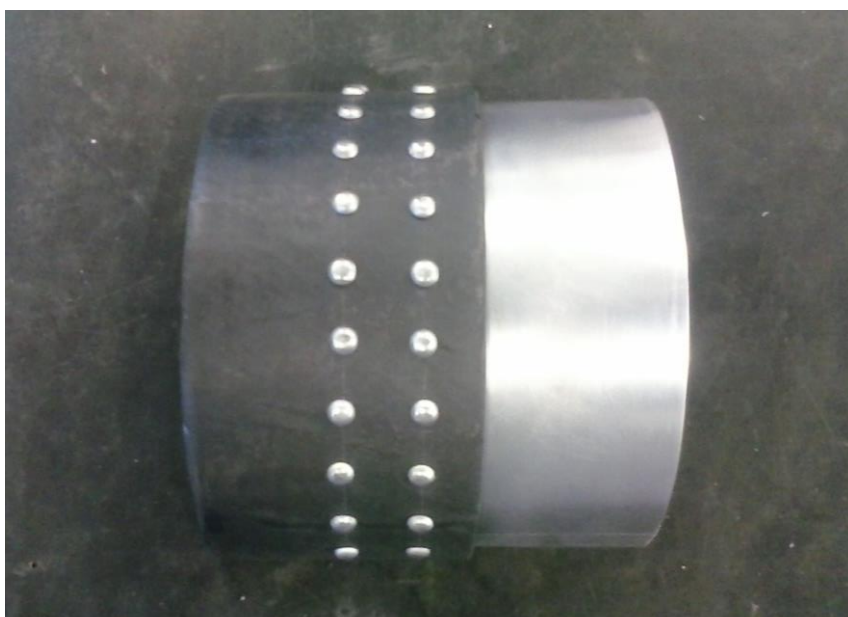
FOTO 1 – Carenagem de Compósito e Alumínio Rebitado (Exercício Avaliação)
